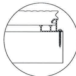
Montageabschluss , letztes WPC-Profil mit Alu-Profil "9541"
