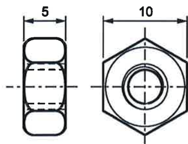
Mutter M6
